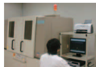
X線回折装置
