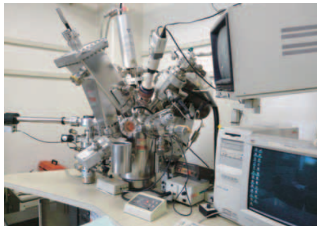
微量元素分析装置 (共同研究イノベーションセンター)
